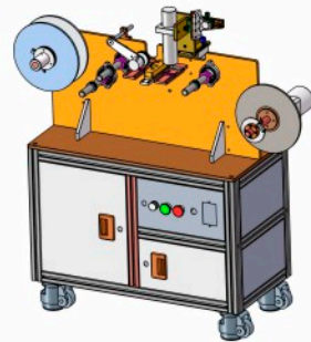
标签回卷机 Label rewinder
